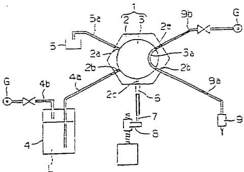
本発明の第一の実施の形態を示す装置構成図
